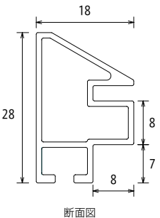
断面図
