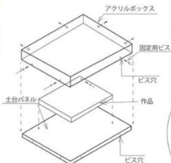
図例：F4 サイズ (サイズによってビス留め数が異なります) ※F10のみ中サン付の土台パネルとなります。
